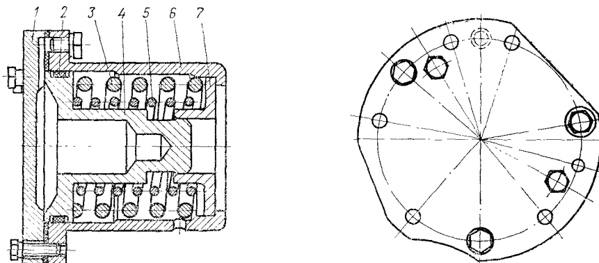
Рис. 45. Гидроаккумулятор гидросистемы трансмиссии трактора Т-150К:
