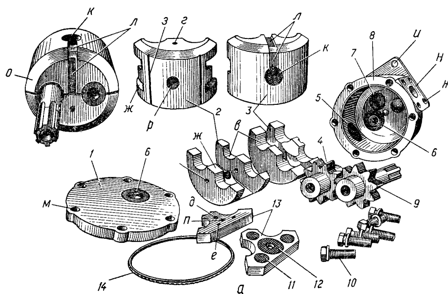
Рис. 4. Шестеренный круглый насос типа НШ-К:
