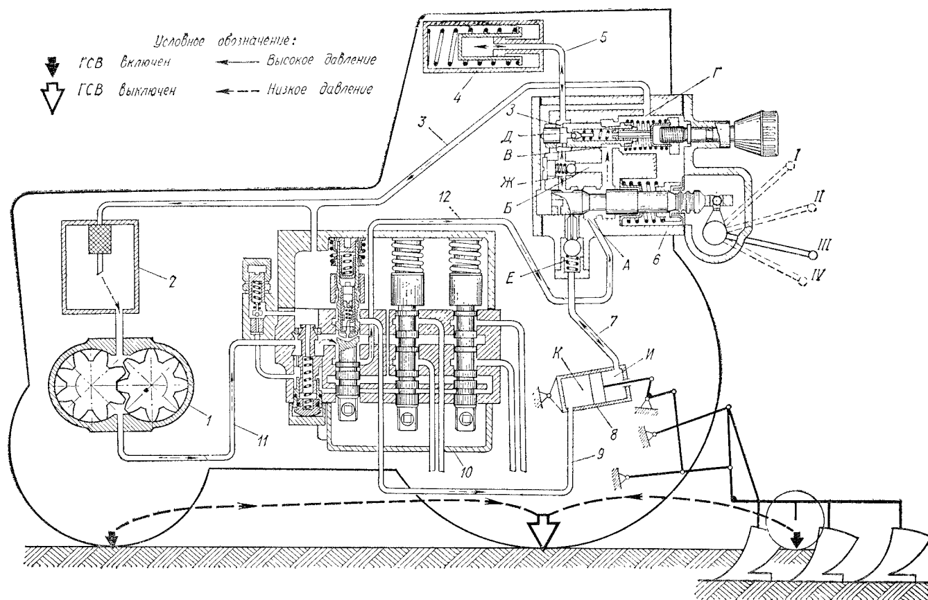
Рис. 31. Схема работы гидравлической системы трактора МТЗ-80 (МТЗ-82) с гидроувеличителем сцепного веса: 1 — насос; 2 — бак для рабочей жидкости; 3, 5, 7, 9, 11 и 12 — трубопроводы, соединяющие агрегаты гидросистемы; 4 — пружинный гидроаккумулятор; 6 — гидроувеличитель; 8 — цилиндр; 10 — распределитель, положение рукоятки гидроувеличителя. I — «Заперто»; II — «Выключен»; III — «Включен»; IV — «Сброс давления»; А, Б, В, Г, Д, Е, Ж, З, И, К — ports.
