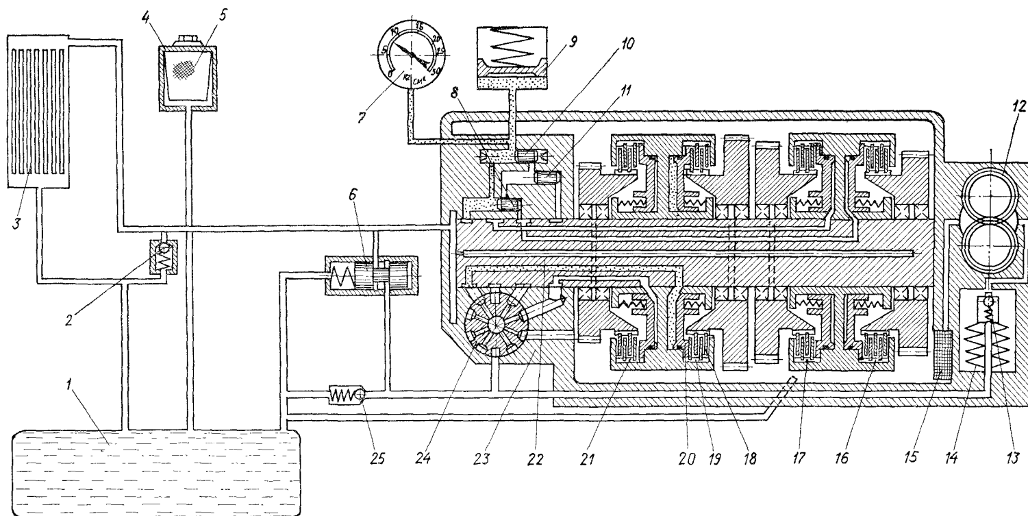
Рис. 43. Схема гидросистемы коробки перемены передач трактора Т-150К:
