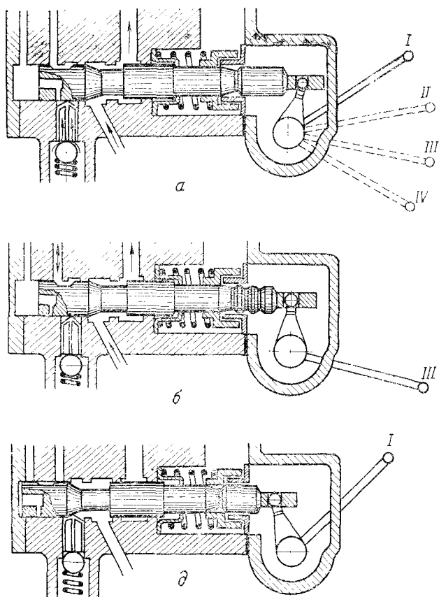
Рис. 33. Положения ползуна, золотника, а также обратного клапана в корпусе гидроувеличителя при зарядке аккумулятора: а — разгрузка от давления; б — ГСВ включен; в — зарядка гидроаккумулятора; г — ГСВ выключен; д — силовой цилиндр закрыт.
