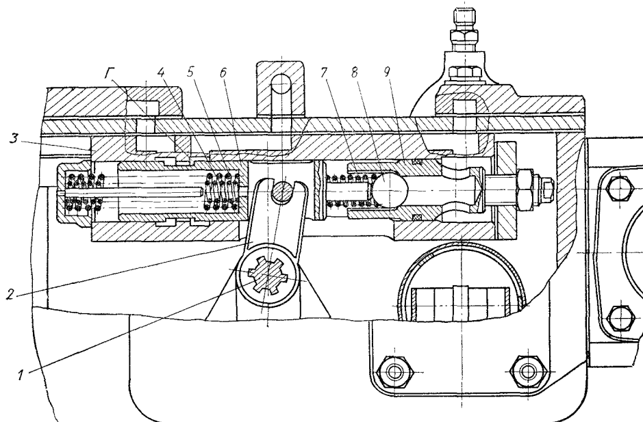
Рис. 57. Клапан плавного снижения давления гидросистемы трансмиссии трактора Т-150:
