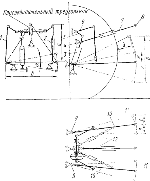
Рис. 1. Схема заднего навесного трехточечного механизма:
