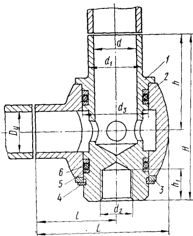
Рис. 22. Поворотное соединение:
