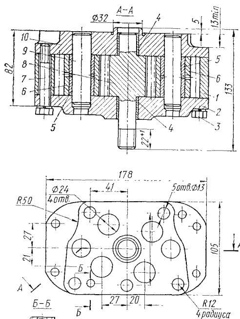
Рис. 9. Насос шестеренный двухсекционный НМШ-125: 1 — корпус; 2 — верхняя крышка; 3 — болт; 4 и 5 — опорные втулки ведущей и ведомой шестерен; 6 — ведомая шестерня; 7 — болты, соединяющие корпус с крышками; 8 — ведущая шестерня; 9 — ось ведомой шестерни; 10 — нижняя крышка; 11 — штифт-фиксатор.
