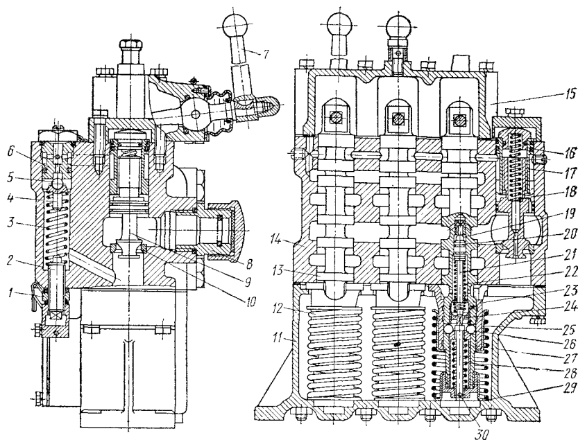
Рис. 13. Распределитель: P150-B3:
