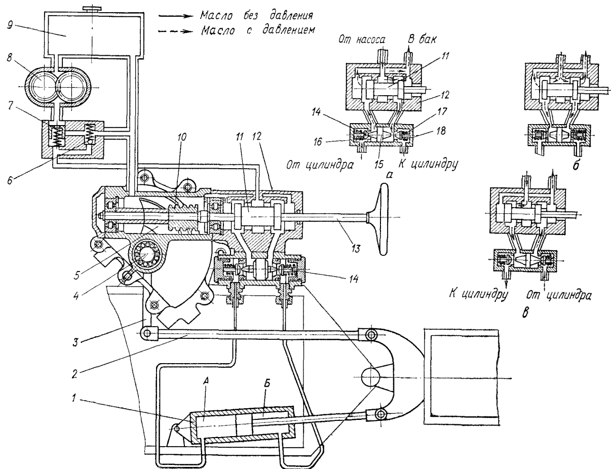
Рис. 49. Схема гидросистемы рулевого управления трактора Т-150:
