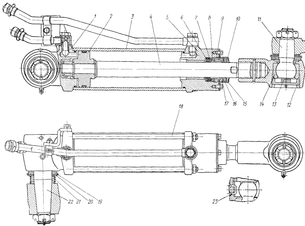
Рис. 52. Гидроцилиндр гидросистемы рулевого управления трактора Т-150К:
