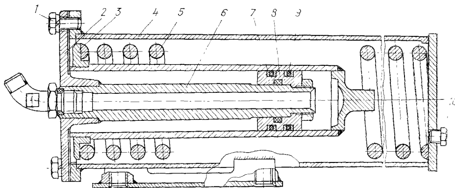
Рис. 32. Пружинный гидроаккумулятор:
