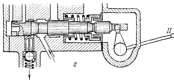
Рис. 33. Положения ползуна, золотника, а также обратного клапана в корпусе гидроувеличителя при зарядке аккумулятора: а — разгрузка от давления; б — ГСВ включен; в — зарядка гидроаккумулятора; г — ГСВ выключен; д — силовой цилиндр закрыт.
