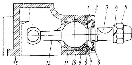
Рис. 12. Узел управления распределителя Р75-ВЗ-А:
